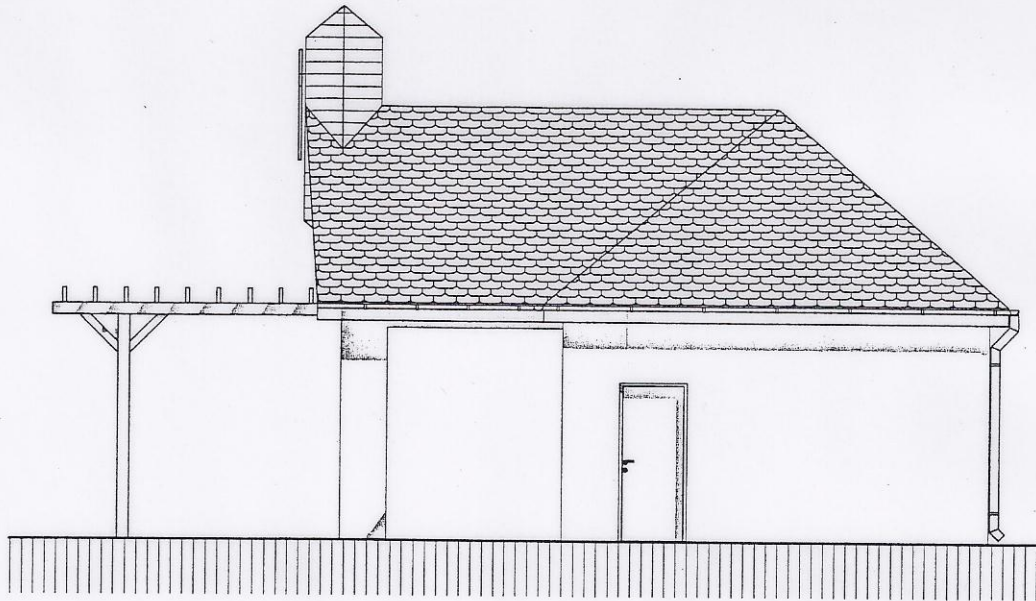
..... HOMLOKZAT M 1:100
