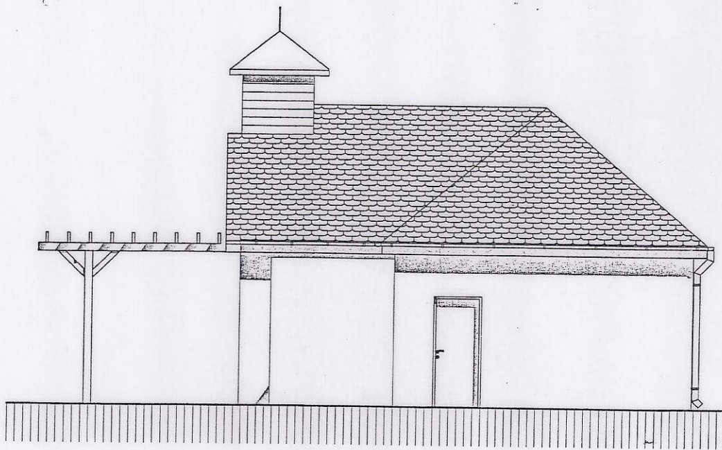
..... HOMLOKZAT M 1:100
